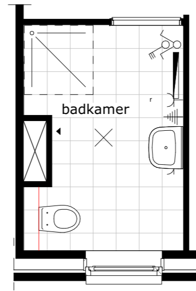
50.52.07 Badkamerindeling D -verplaatsen toilet,
