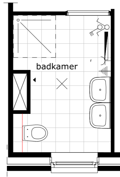
50.52.06 Badkamerindeling C -verplaatsen toilet -dubbele wastafel
