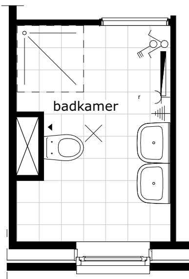
50.52.08 Badkamerindeling E -dubbele wastafel
